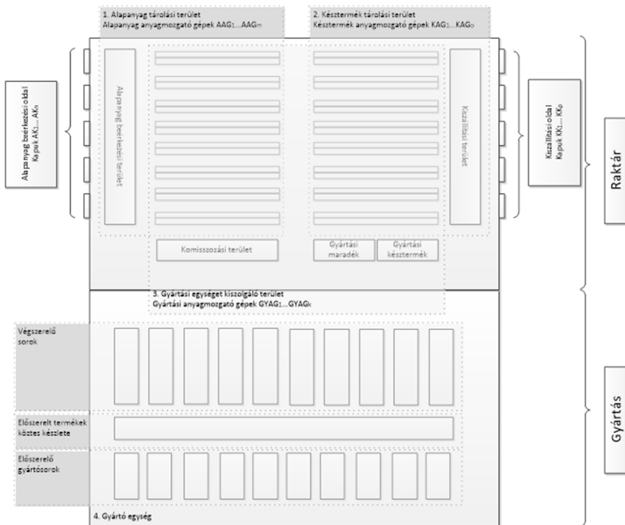
9. ábra Raktári elrendezési modell [saját szerkesztés]
