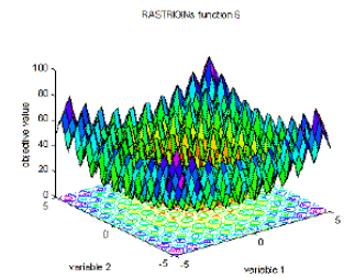
34. ábra: Rastrigin függvény
