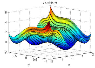
33. ábra: Hatpúpú teve függvény
