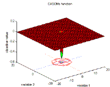
35. ábra: Easom tesztfüggvény
