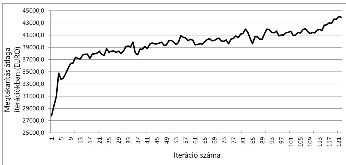
42. ábra: Optimalizálási folyamat konvergenciagörbéje
