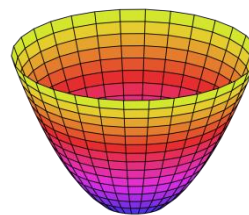
29. ábra: Parabola függvény
